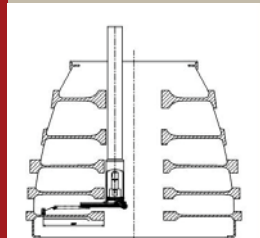
Abb. 1: Teleskop-Achse für die Prüfung des Spool 2 - 6
