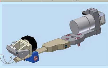
Abb. 3: kompakter Prüfkopfmanipulator mit Spiegelvorsatz
