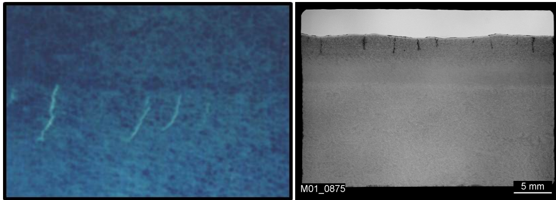
Abbildung 4. Risse in den in dem Vorhaben untersuchten plattierten Testkörpern: Unterplattierungsrisse. Links: Ergebnisse einer fluoreszierenden Magnetspulverprüfung. Rechts: Schliffbild.
